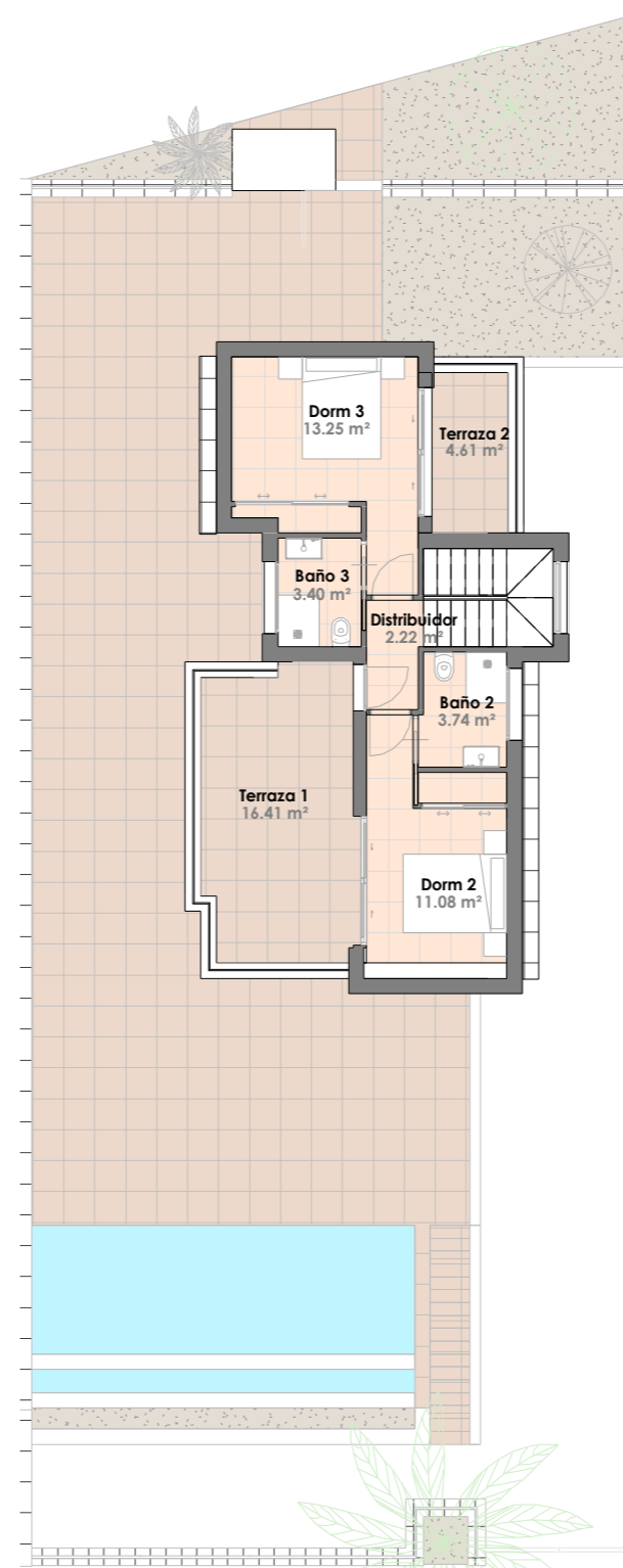
Planta Primera
