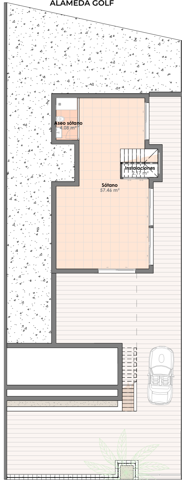
Planta Sótano
