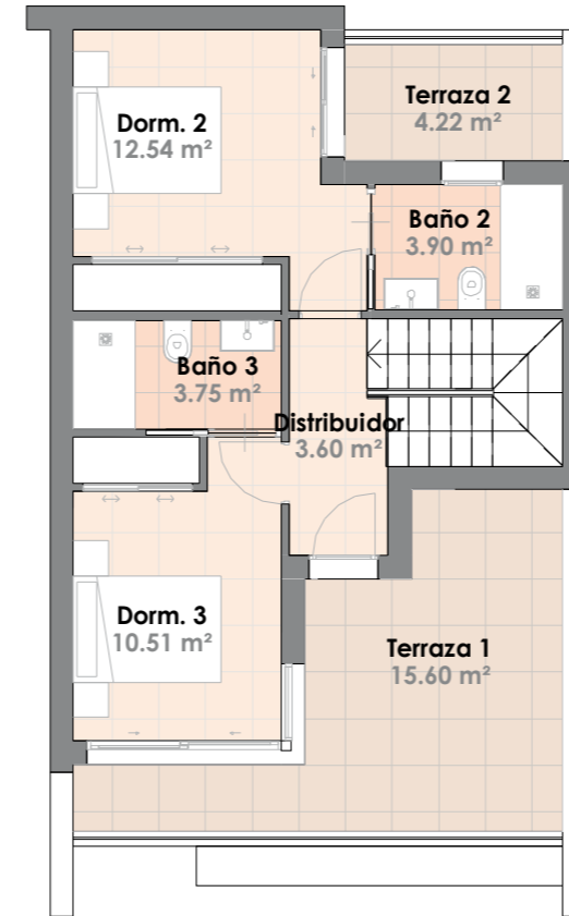
Planta Primera
