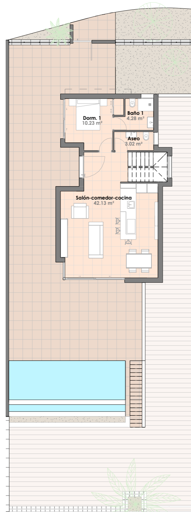
Planta Baja
