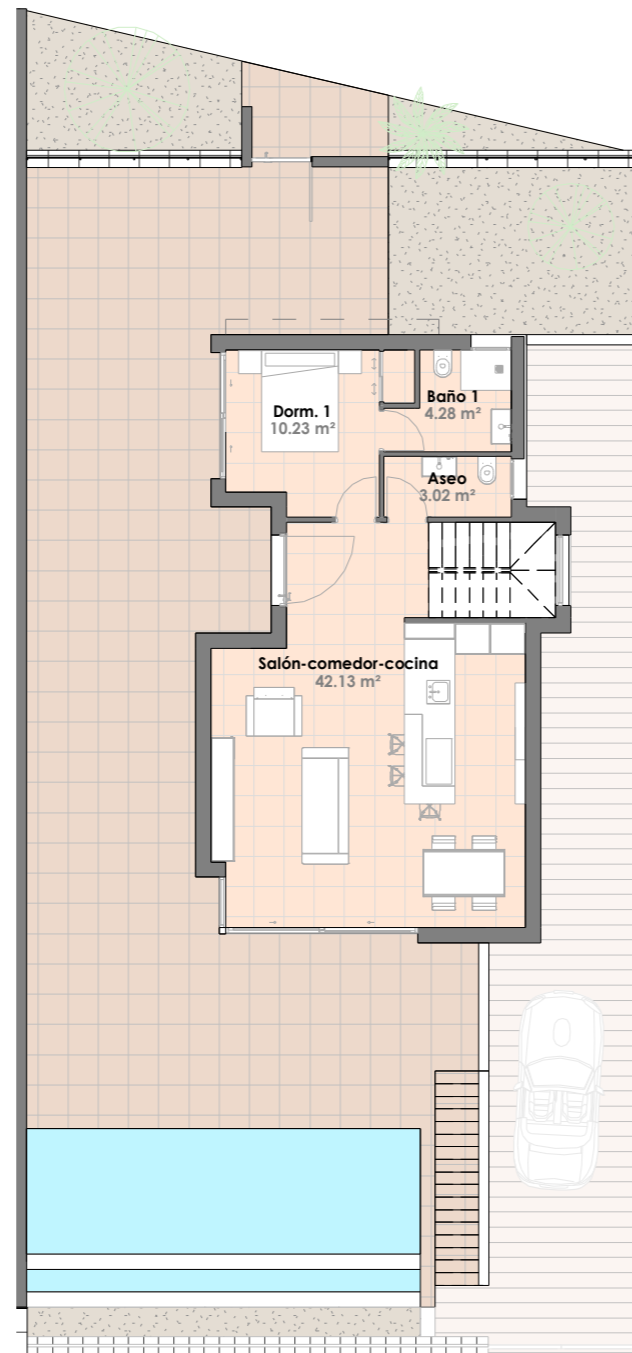
Planta Baja
