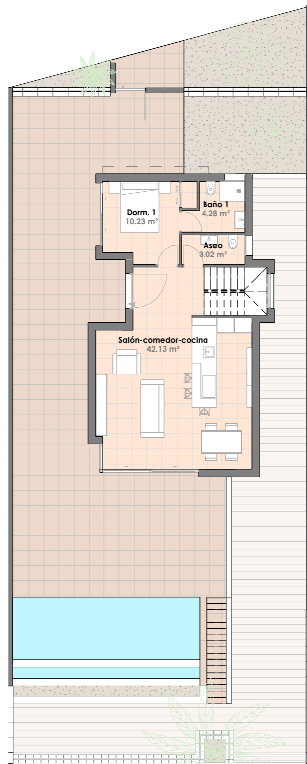
Planta Baja
