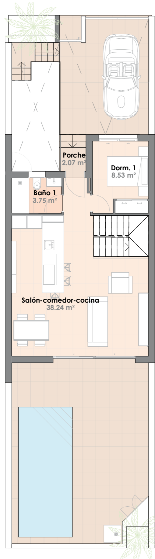
Planta Baja
