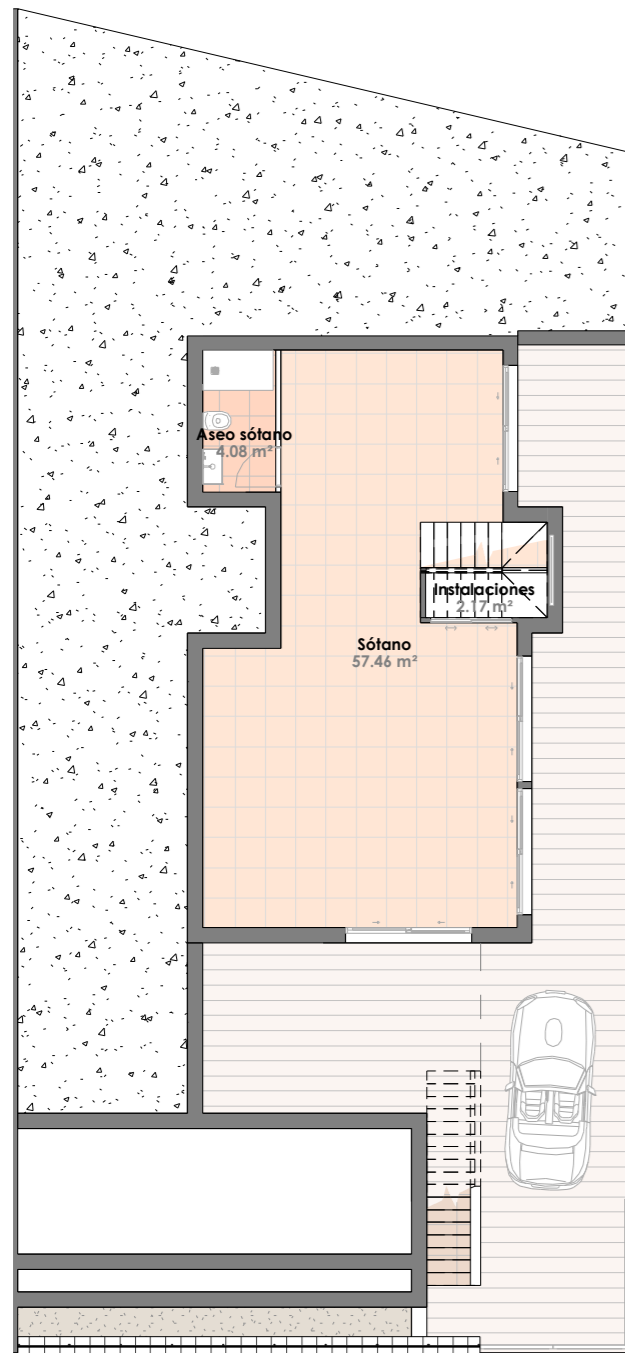
Planta Sótano
