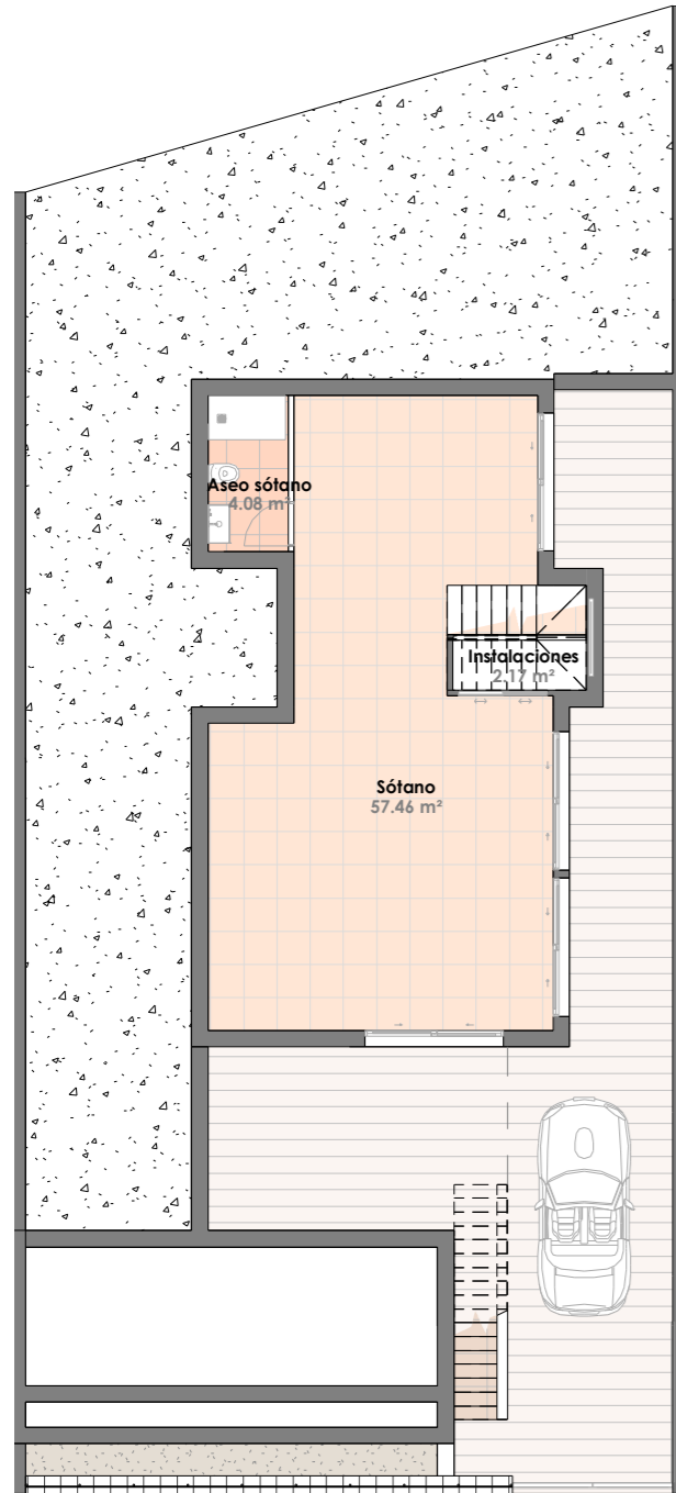
Planta Sótano
