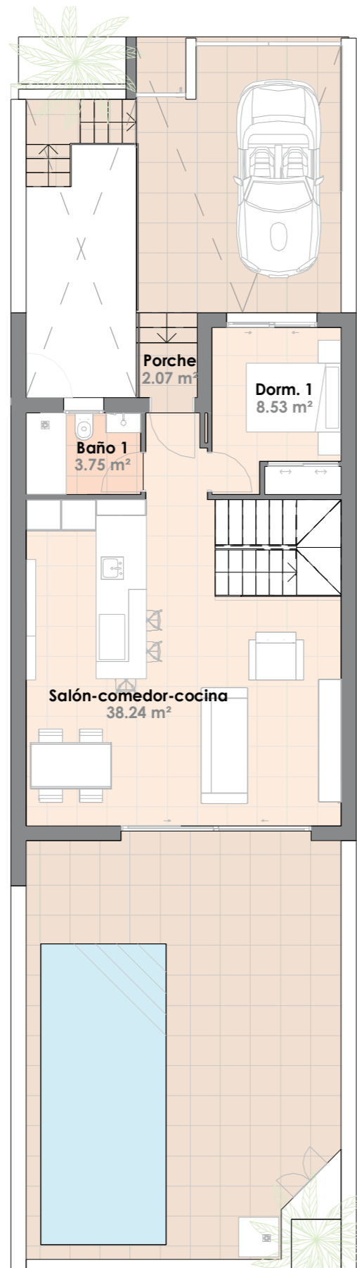
Planta Baja
