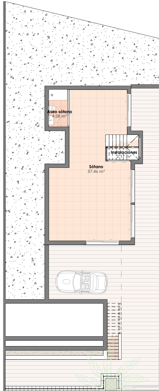
Planta Sótano
