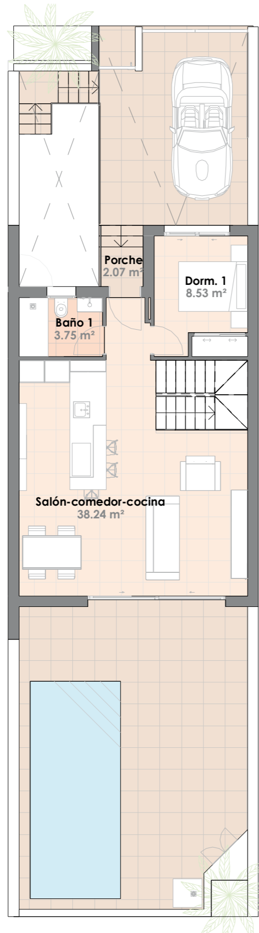
Planta Baja
